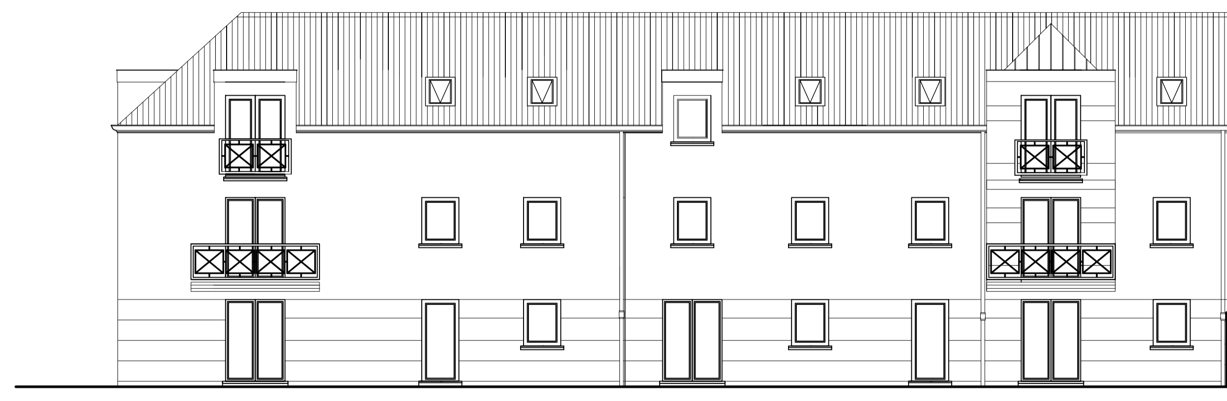
Batiment B1 et B2 : Façade sur Jardin
